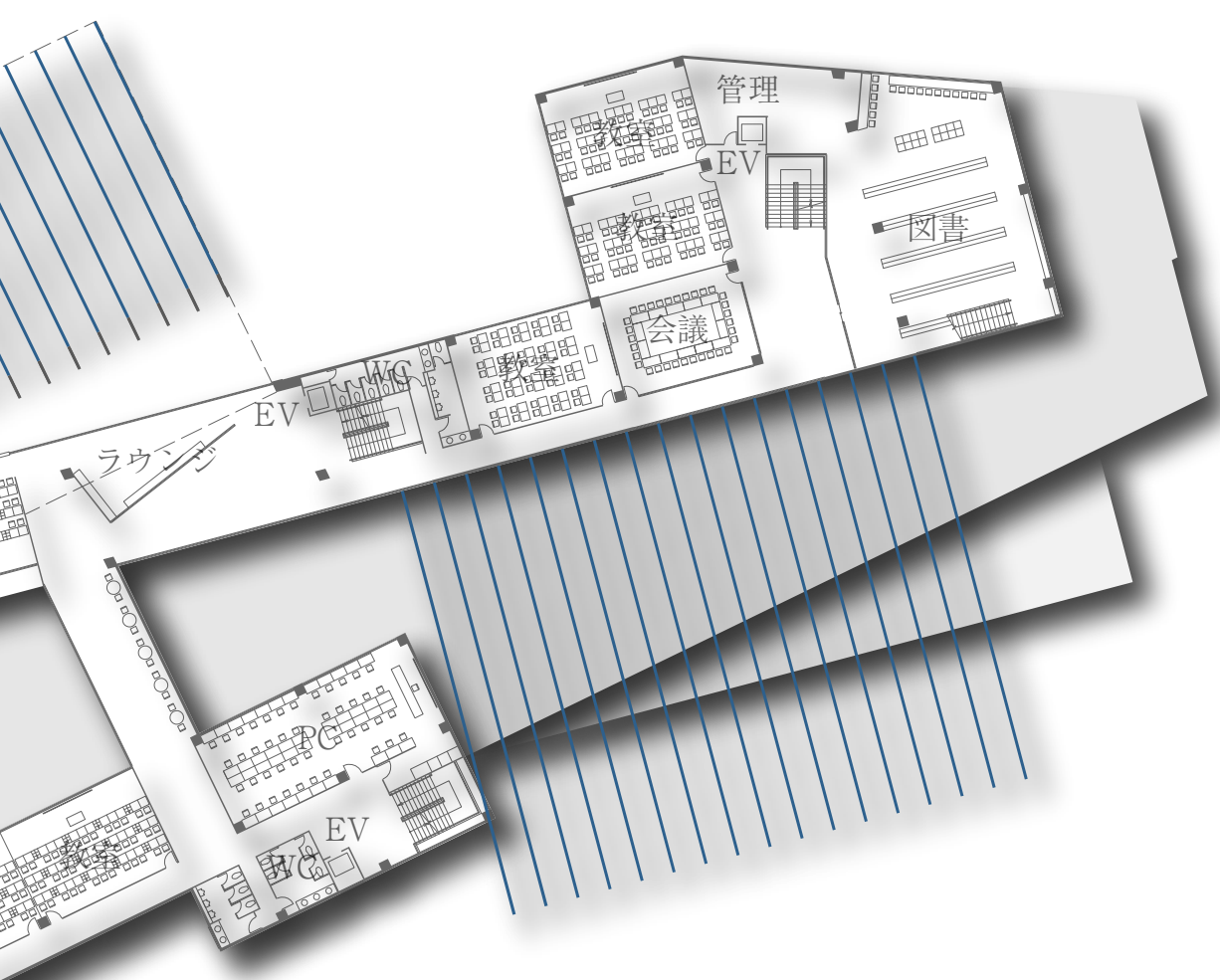
平面図 4階 S : 1/500
