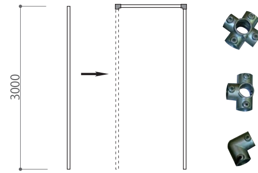
②単管パイプ+ジョイント
