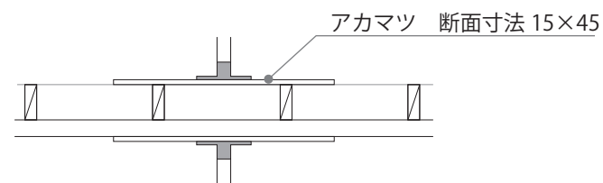
⑤上部パネルと支柱の接合部
