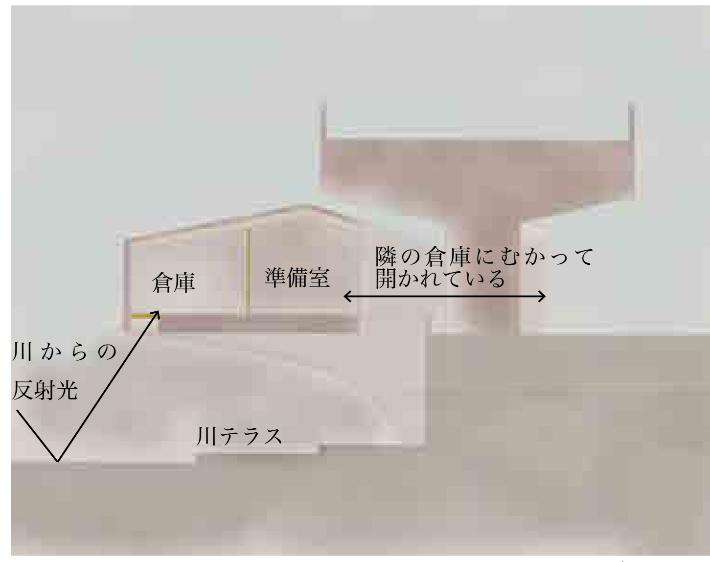
断面図 S=1:200
