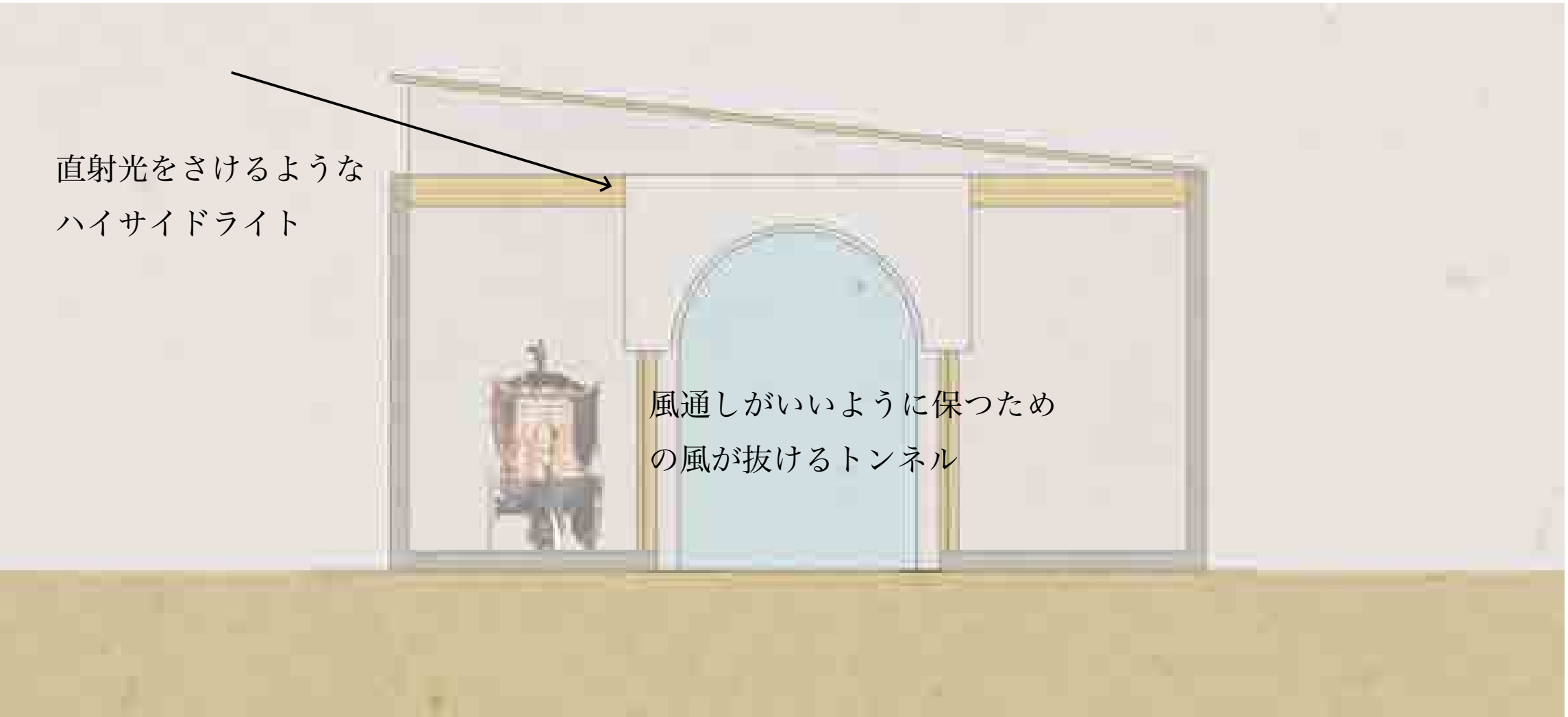
断面図 S=1:100
